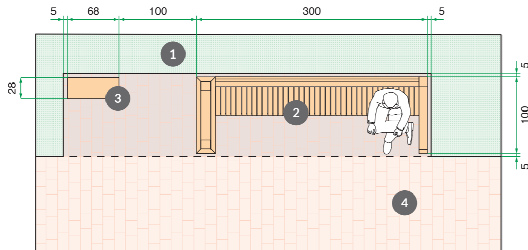
300 x 100 x 245 cm z bocznymi ściankami
