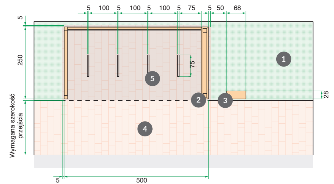
Wiata rowerowa 500 x 250 cm
