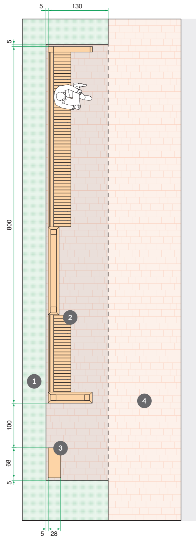
Wiata przystankowa 800 x 130 x 245 cm z bocznymi ściankami
