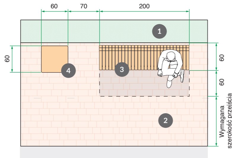
Ławka z oparciem i pojemnikiem na zielen na ciągu pieszym
