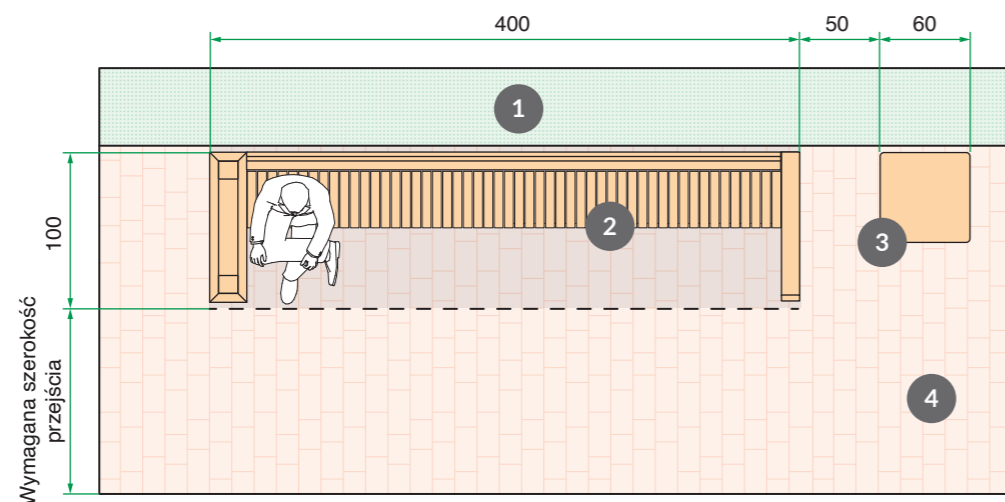
400 x 100 x 245 cm z bocznymi ściankami
