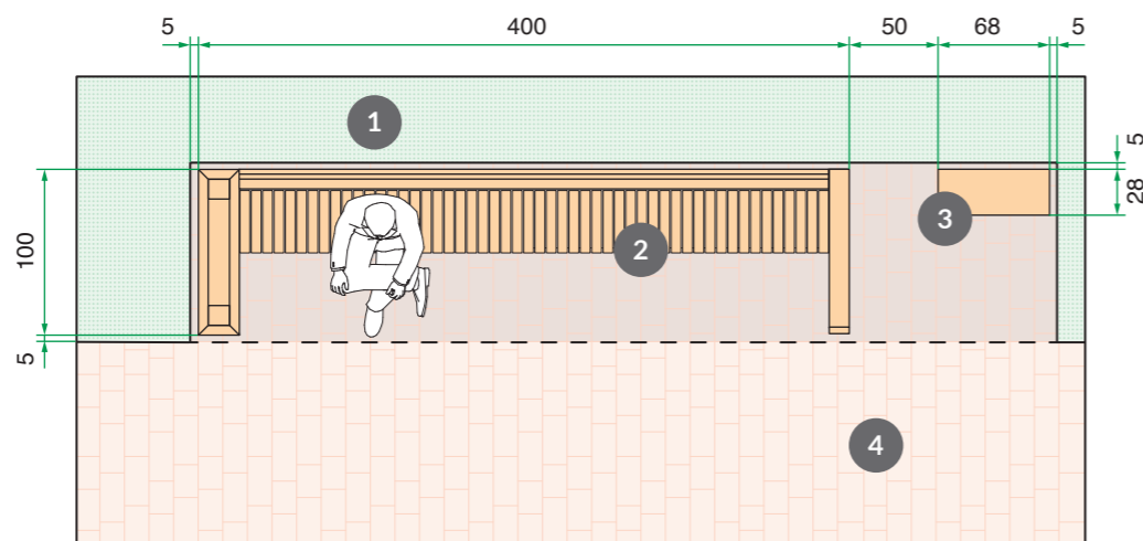
400 x 100 x 245 cm z bocznymi ściankami
