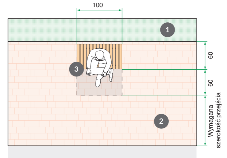
Ławka bez oparcia poza ciągiem pieszym
