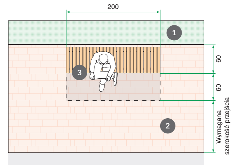
Ławka bez oparcia na ciągu pieszym
