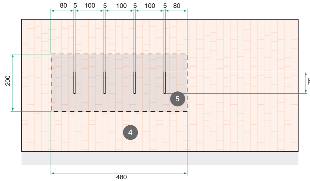
Stojaki rowerowe w strefie ruchu pieszego
