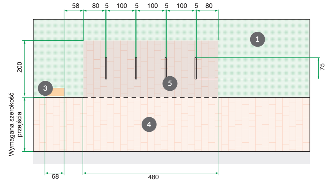
Stojaki rowerowe po za ciągiem pieszym
