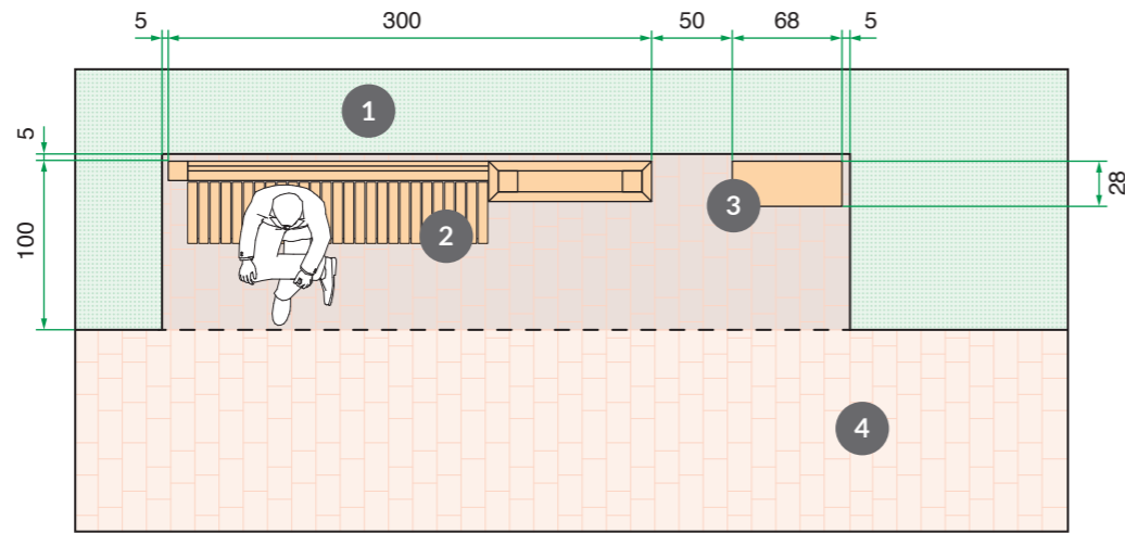
300 x 100 x 245 cm bez ścian bocznych
